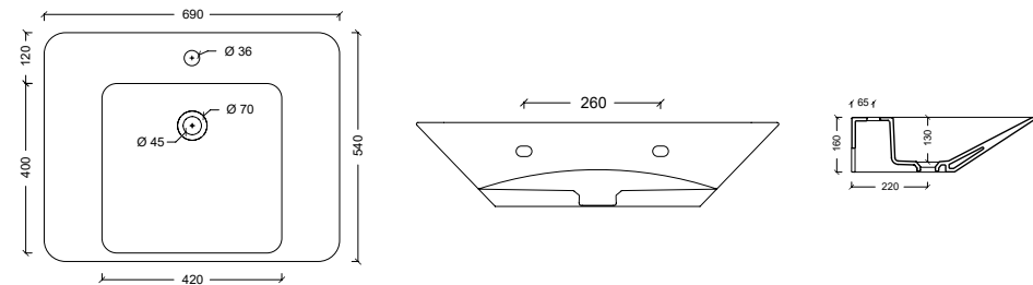
26130101 Lavabo EDGE 59X54 THIN
