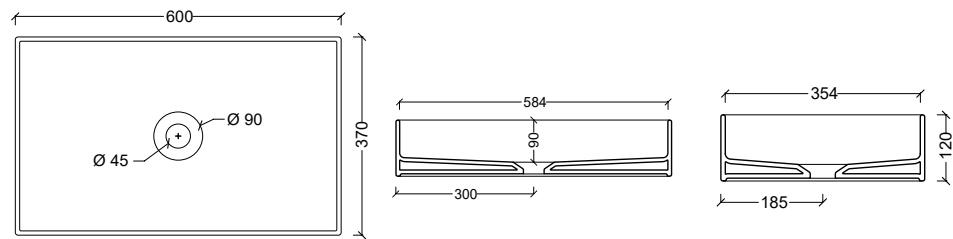
31140101 Lavabo HIDE CIRCLE
