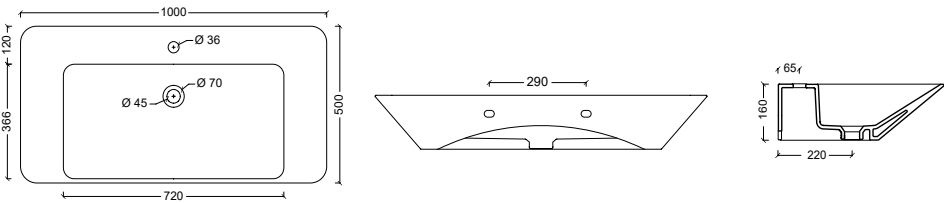
26160101 Lavabo EDGE 80X50
