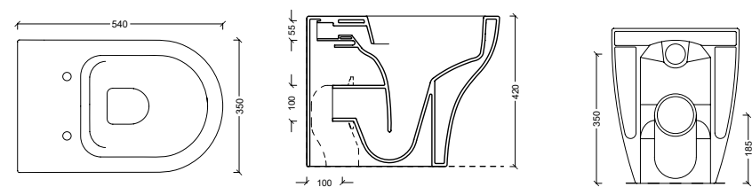
32210101 Bidet UNICA
