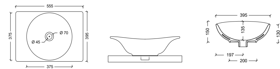
29190101 Lavabo JOKER RETTANGOLARE
