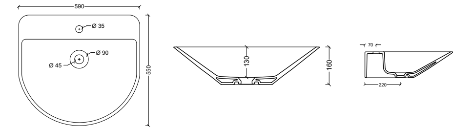
26200101 Lavabo EDGE ROUND
