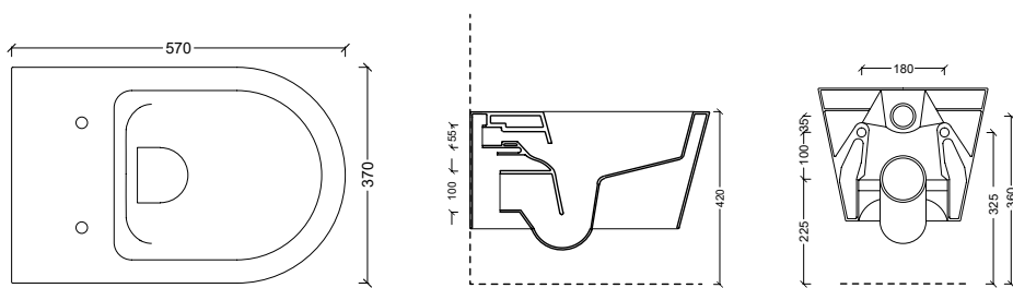
31170101 Vaso sospeso HIDE ROUND
