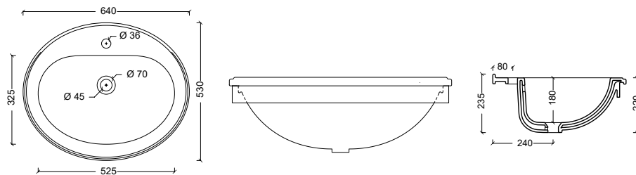
500502 Lavabo DECOR 63
