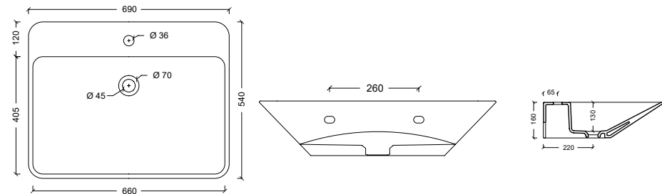
26150101 Lavabo EDGE 69X54 THIN
