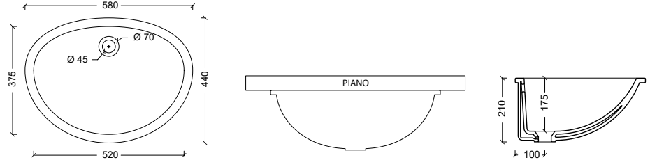
27190401 Lavabo TIPO
