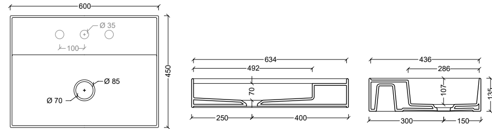
31230101 Lavabo sospeso e appoggio 60 x 45
