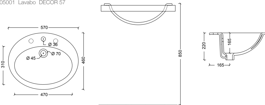
5005001 Lavabo DECOR 57
