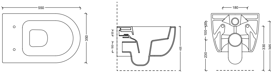
32240101 Vaso sospeso UNICA 55
