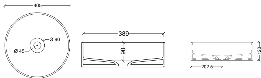
31140101 Lavabo HIDE CIRCLE
