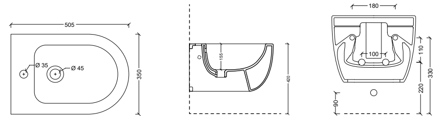
32230101 Bidet sospeso UNICA 50
