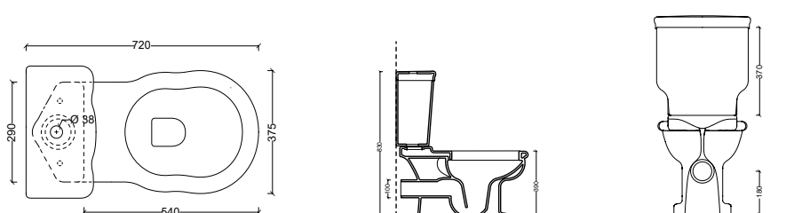
28290101 Vaso Monoblocco BOHEME scarico a parete
