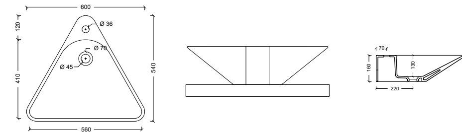
26210301 Lavabo EDGE TRIO
