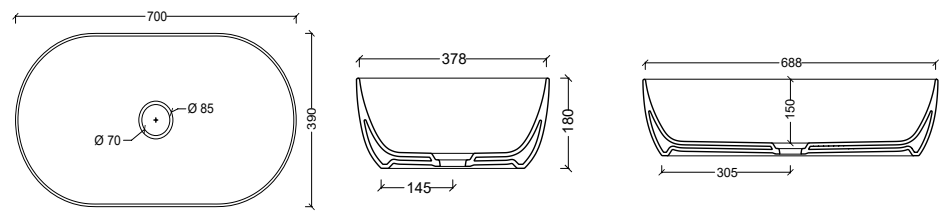
32120101 Lavabo UNICA 55X35
