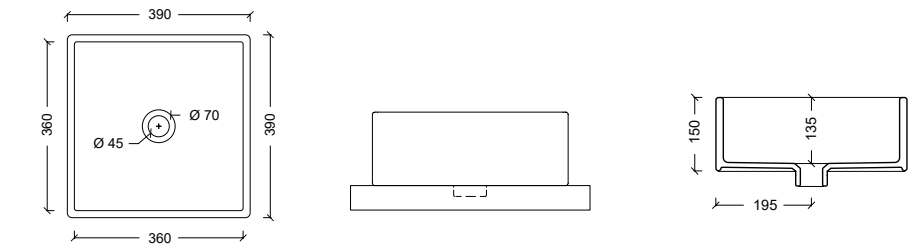
29110101 Lavabo JOKER QUADRATO
