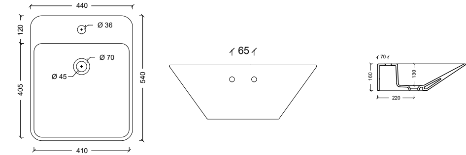
26100301 Lavabo EDGE 44X44
