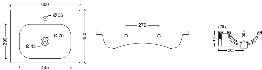
23100601 Lavabo NEAT 60
