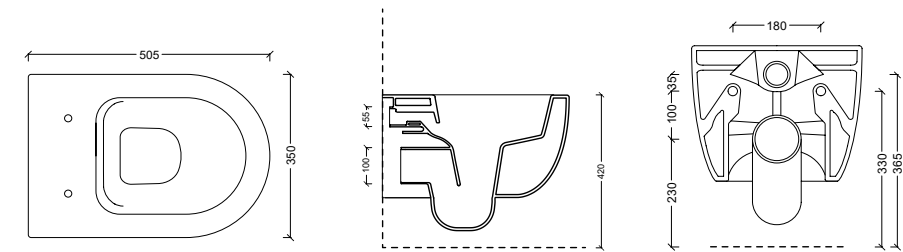
32220101 Vaso sospeso UNICA 50
