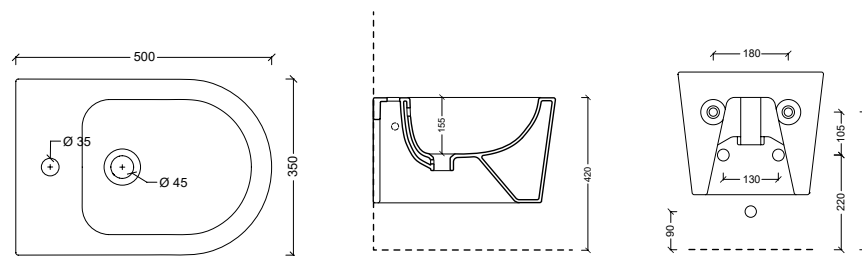
22310101 Bidet sospeso FORM SQUARE
