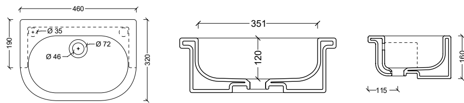
22130501 Lavabo FORM 46 ROUND SEMINCASSO
