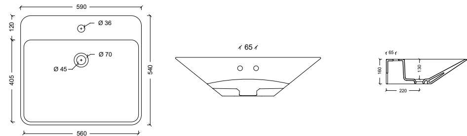
26200101 Lavabo EDGE ROUND
