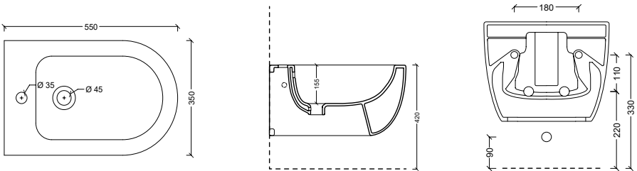
32250101 Bidet sospeso UNICA 55
