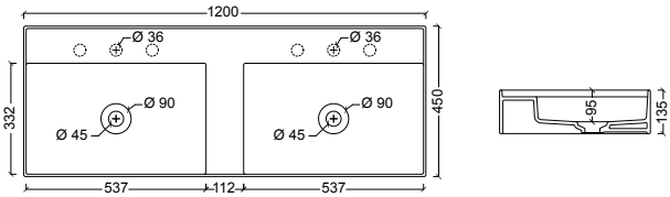
31260101 Lavabo sospeso e appoggio HIDE 120 X 45
