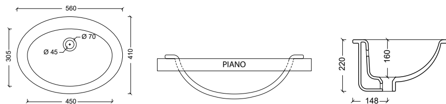
500500 Lavabo DECOR 56
