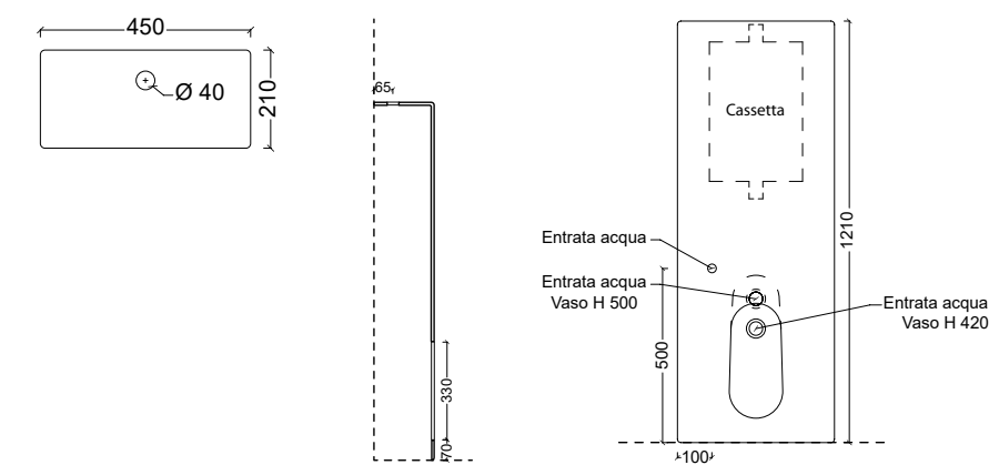
22330101 FORM PLUS
