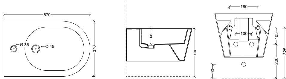
31180101 Bidet sospeso HIDE ROUND
