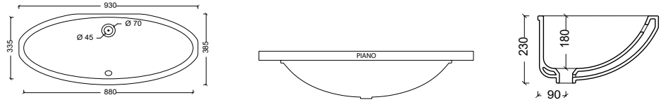
27130401 Lavabo FILO 70
