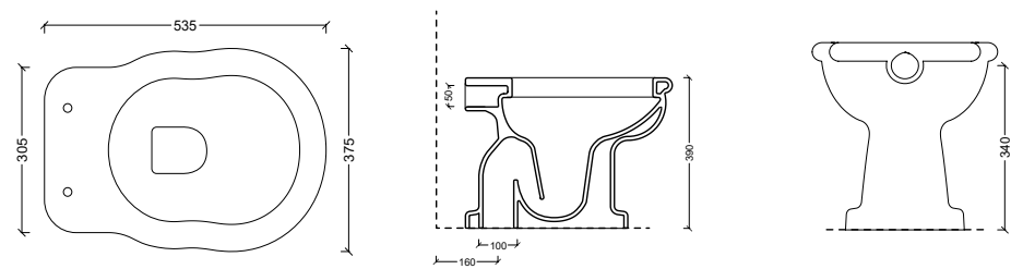
28210101 Vaso a terra BOHEME scarico a parete
