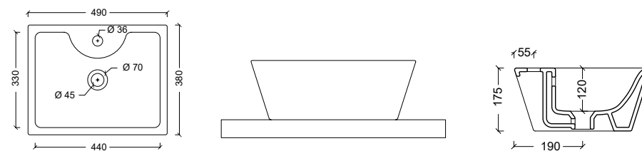
24110301 Lavabo TULIP BIG
