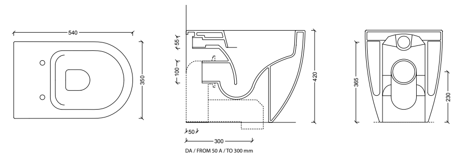
22240101TR Vaso a terra FORM SQUARE TRASLATO RIMLESS
