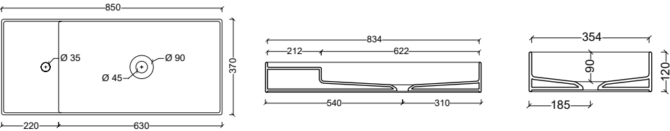
31110101 Lavabo HIDE 65 X 40
