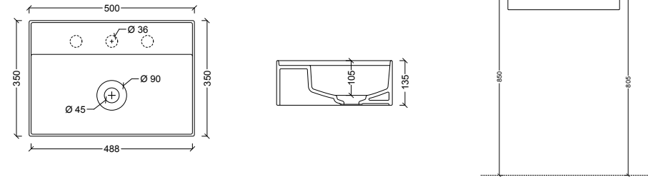
31100101 Lavabo HIDE 85 x 37
