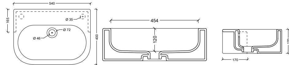
22110501 Lavabo FORM SEMINCASSO 54
