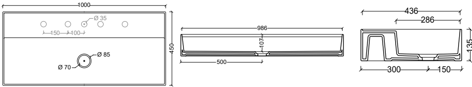
31240101 Lavabo sospeso e appoggio HIDE 80 X 45
