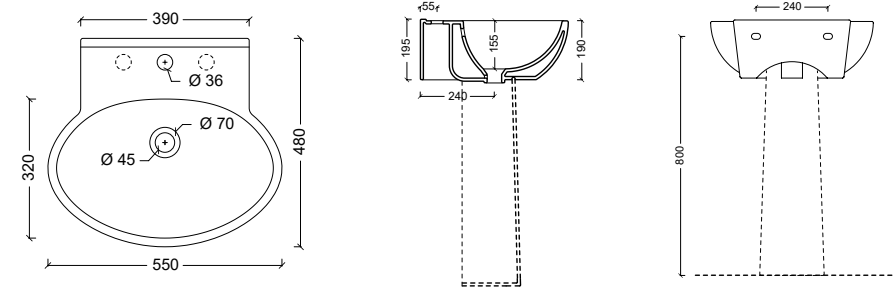
30210101 COLONNA PER LAVABO
