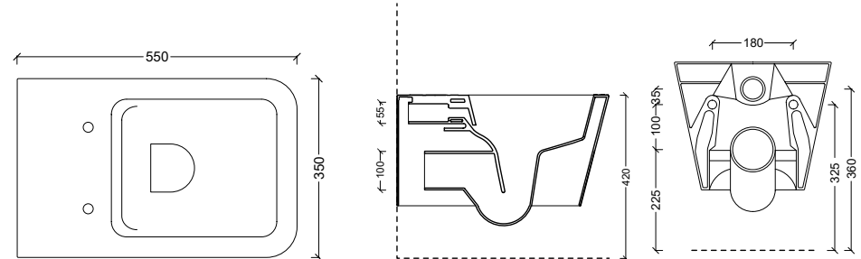
31210101 Vaso sospeso HIDE SQUARE
